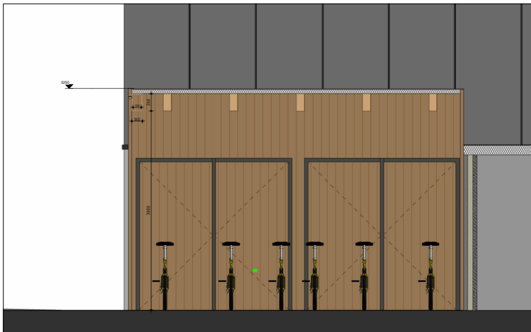
Figuur 3 In het bruin de fietsenstalling met daarboven op de ingebouwde nestkasten. Er wordt ook één nummerstijl geplaatst. Bron: aanvullende informatie van 28 november 2025
