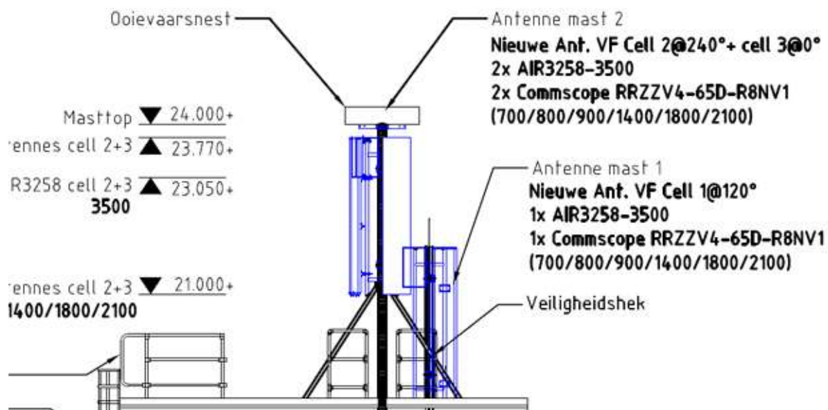
Figuur 7.2. Vooraanzicht en ligging telecommast op gebouw (Ericsson, 2026).
